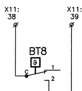
Obr. č. 13 Připojené termostatu čerpadla BT 8 pro kotel VIADRUS GRAND G 36
