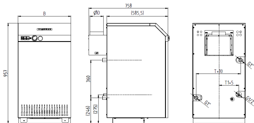
Obr. č. 14 Napojení na otopný systém a montáž přerušovače tahu
