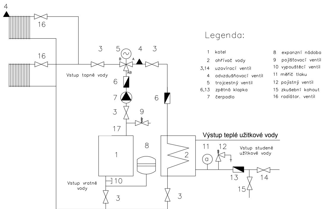
Obr. č. 10 Doporučené schéma zapojení pro přednostní ohřev TV
