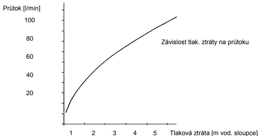
Obr. č. 11 Charakteristika trojcestného ventilu Honeywell V 4044F
