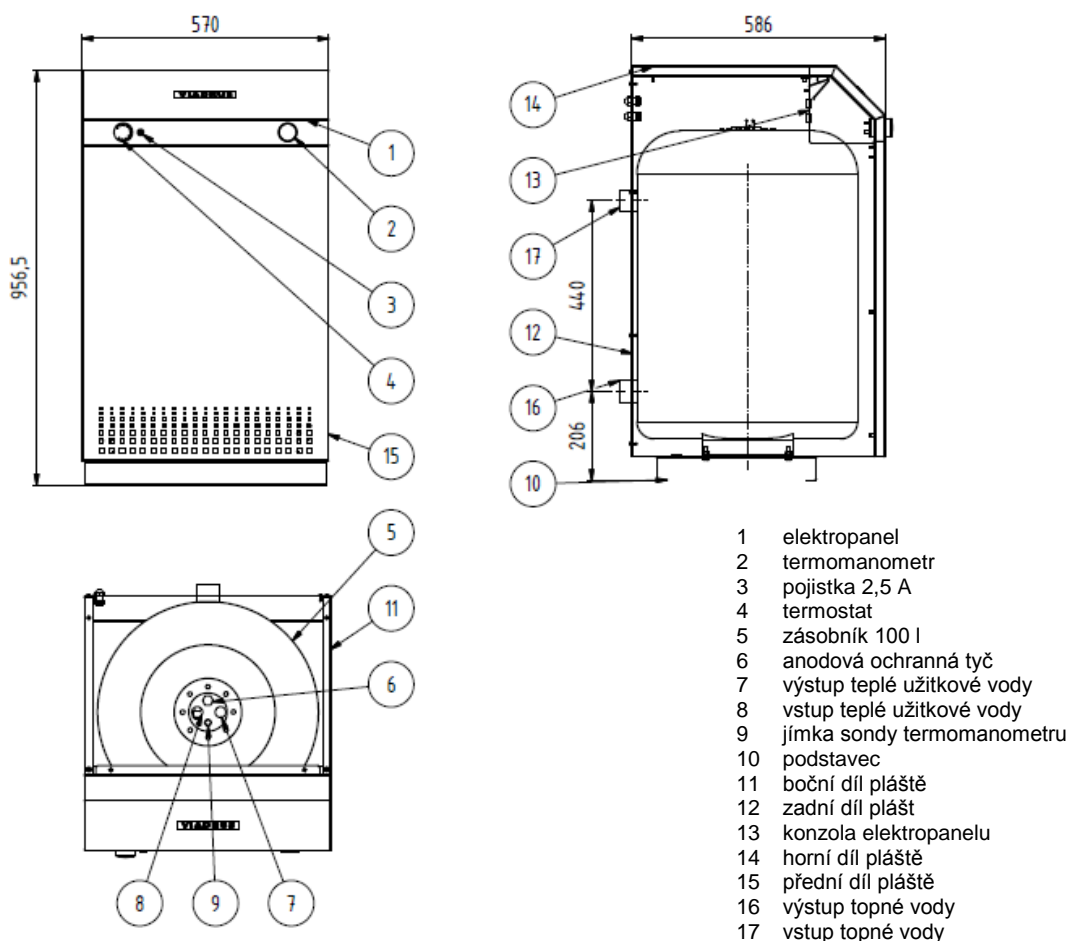
Obr. č. 9 Schéma ohřívače VIADRUS OV 100 L (míry v mm)
