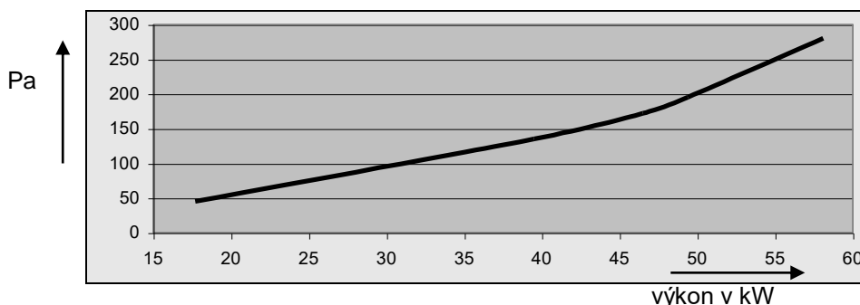
Obr. č. 1 Hydraulická ztráta kotlového tělesa
