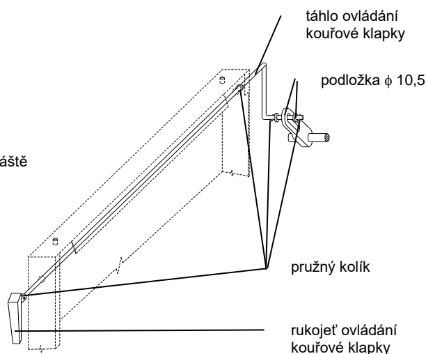
Obr. č. 8 Ovládání kouřové klapky
