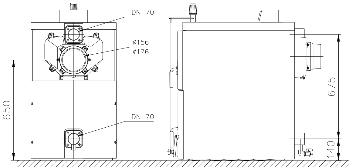
Obr. č. 6 Připojovací rozměry kotle VIADRUS HERCULES U 22
