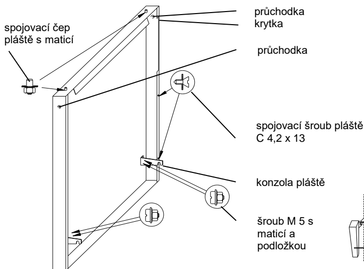
Obr. č. 7 Boční díl pláště
