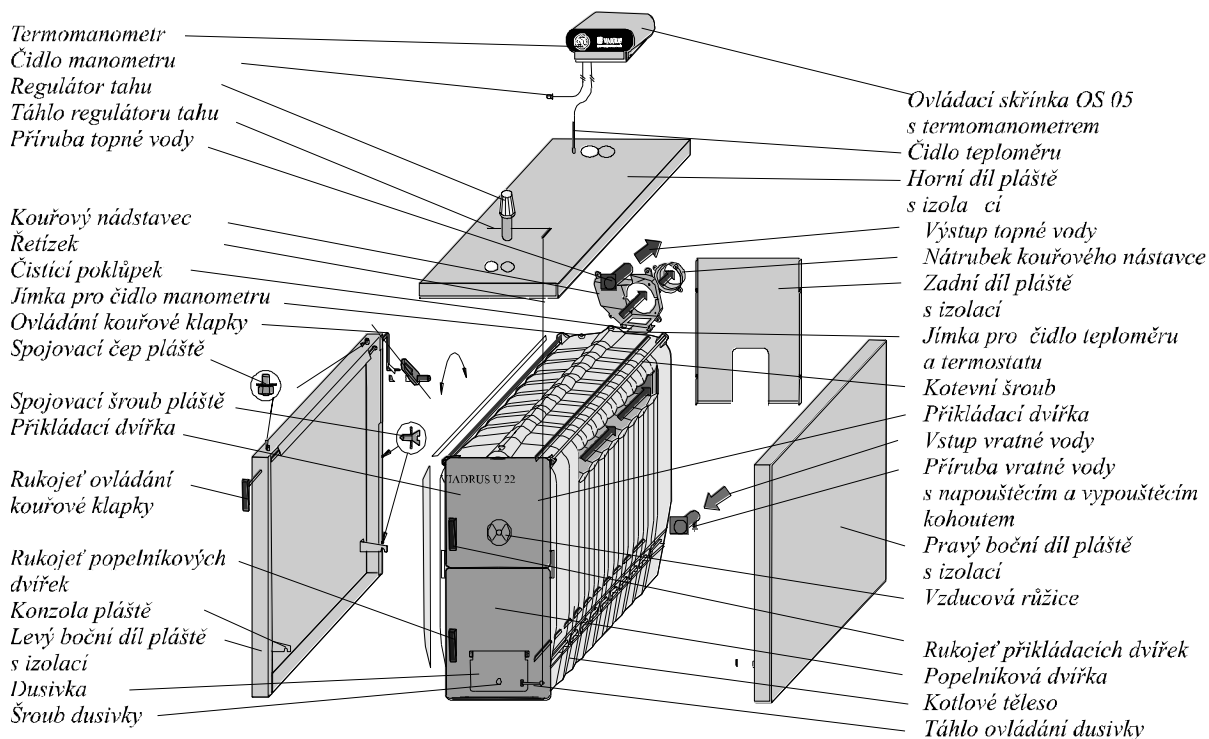
Obr. č. 9 Sestava pláště kotle
