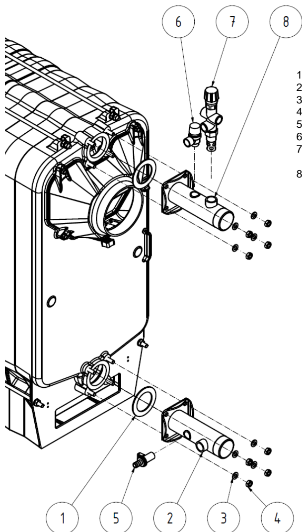
Obr. č. 10 Instalace kotlového tělesa
