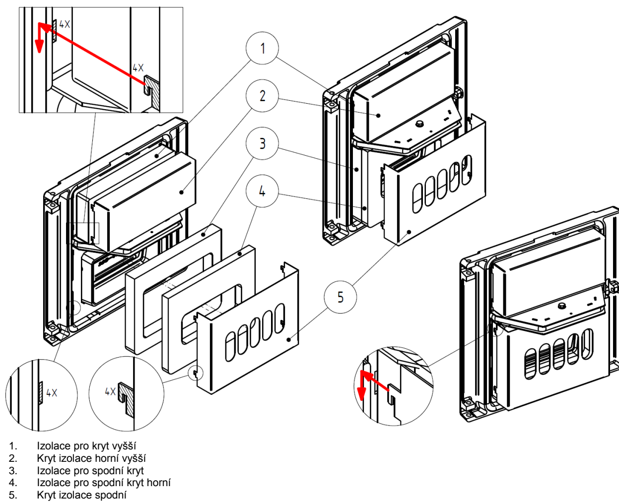
Obr. č. 20 Montáž izolací příkládacích dveří
