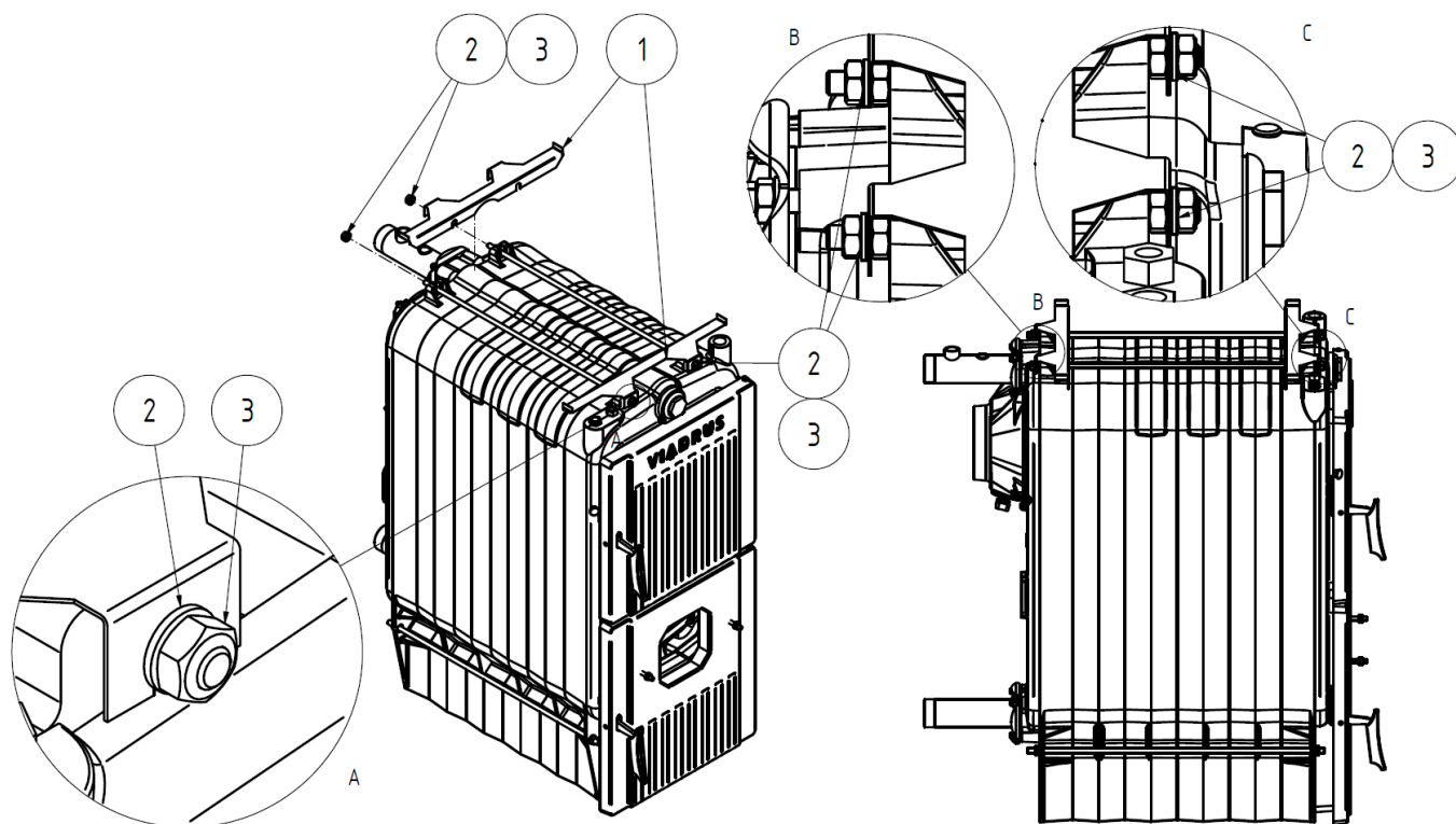
Obr. č. 15 Montáž konzolí pláště
