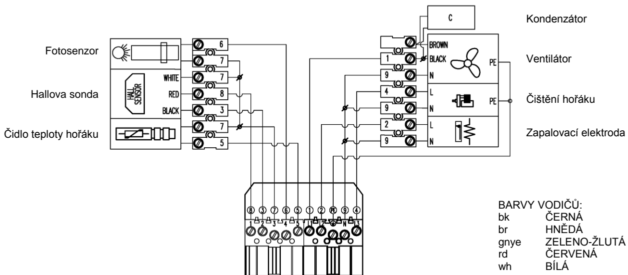
Obr. č. 28 Schéma zapojení hořáku M mini, M mini 35 (čistitelný typy)
