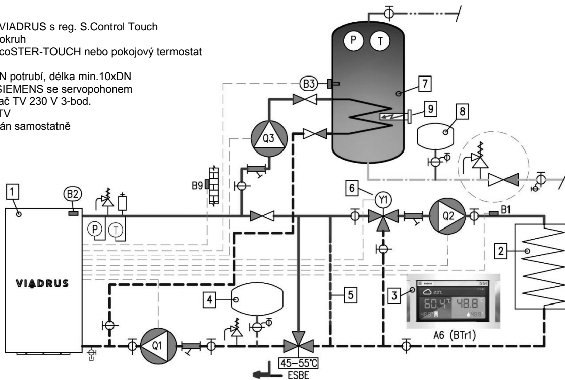
Obr. č. 25 Varianta se směšovaným topným okruhem a s ohřevem TV
