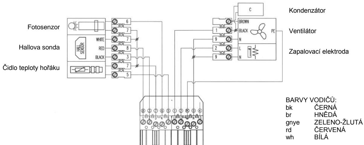
Obr. č. 27 Schéma zapojení hořáku Hybrid mini, Hybrid 35
