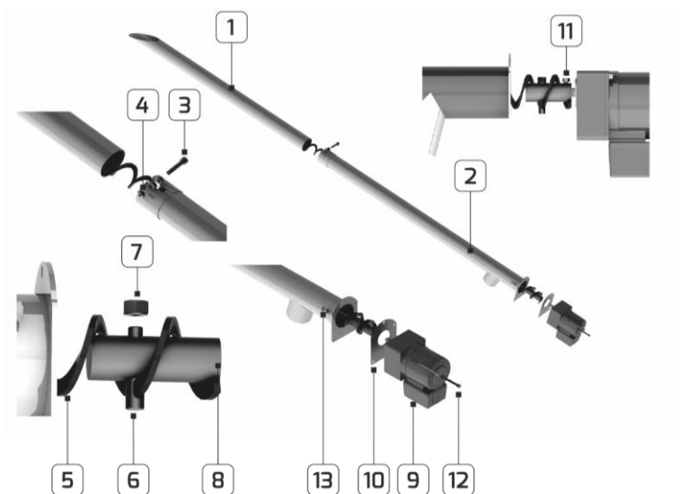
Obr. č. 22 Podavač paliva
