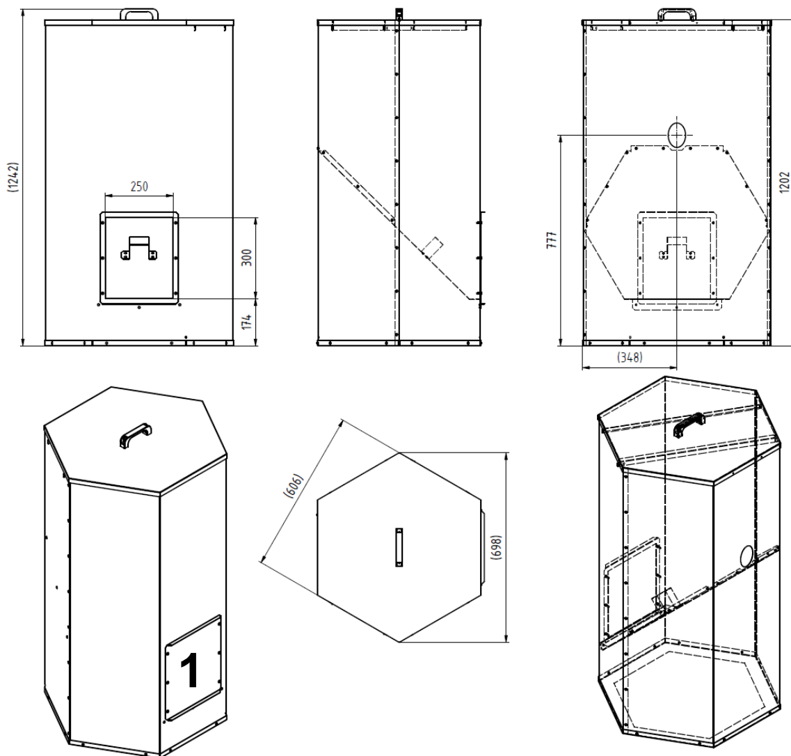
Obr. č. 21 Zásobník paliva (není součástí dodávky)
