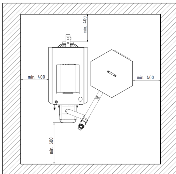
Obr. č. 9 Umístění kotlů v kotelně
