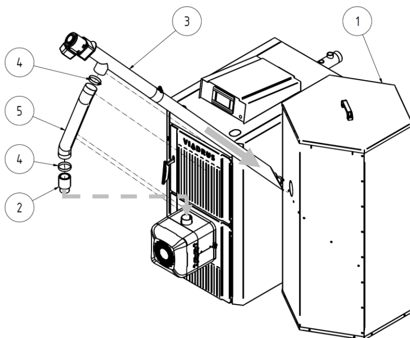
Obr. č. 24 Montáž podavače paliva na kotel
