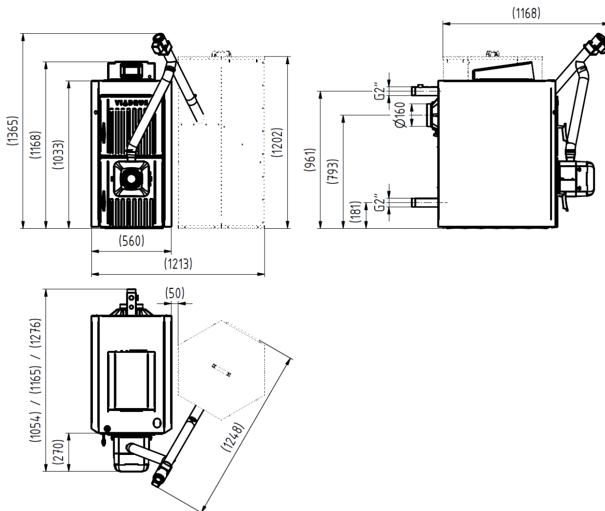
Obr. č. 1 Hlavní rozměry kotle
