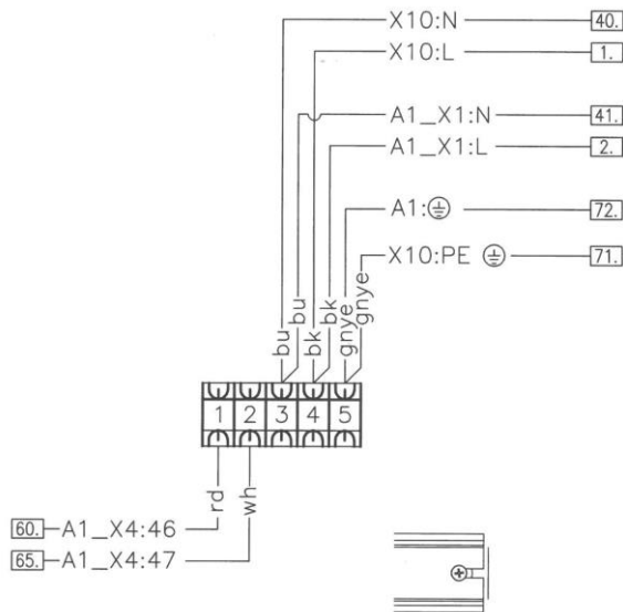
Obr. č. 40 Schéma zapojení
