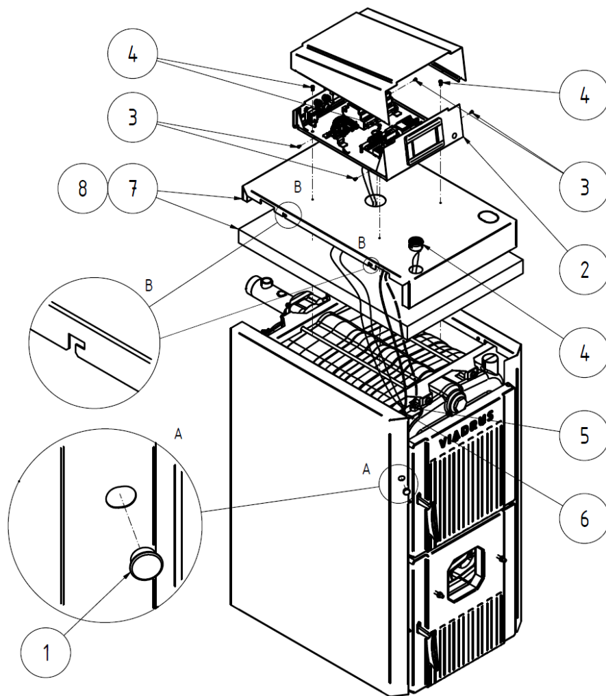
Obr. č. 17 Montáž horního dílu pláště
