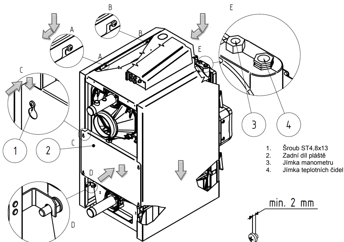
Obr. č. 18 Montáž zadního dílu pláště a nasunutí horního dílu pláště
