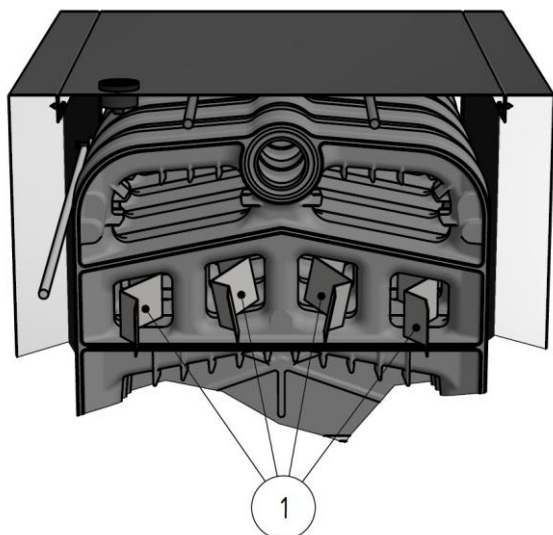
Obr. č. 14 Umístění turbulátorů v kotli
