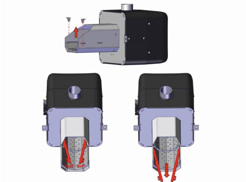
Obr. č. 35 Postup při vytažení ohniště hořáku
