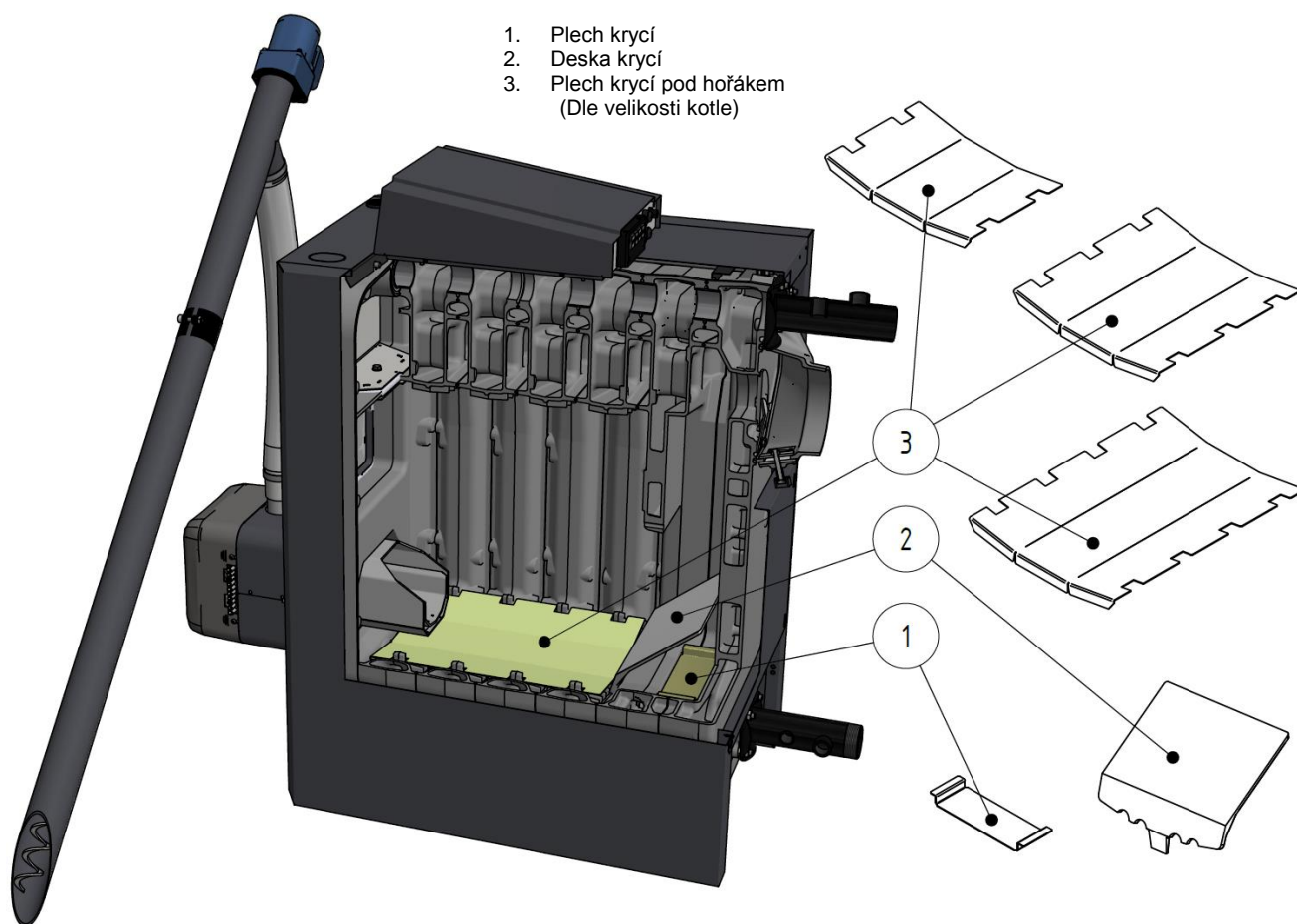
Obr. č. 13 Umístění tvarovek do spalovací komory kotle VIADRUS U22 Economy
