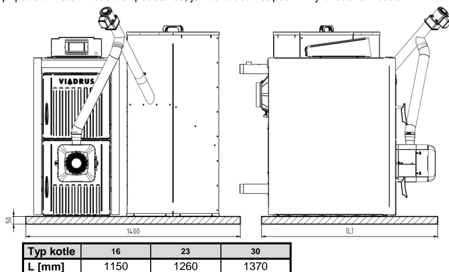
Obr. č. 7 Rozměry podezdívky
