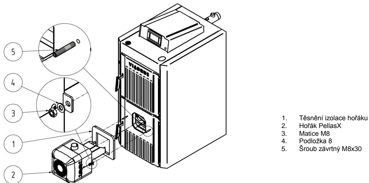
Obr. č. 19 Montáž hořáku
