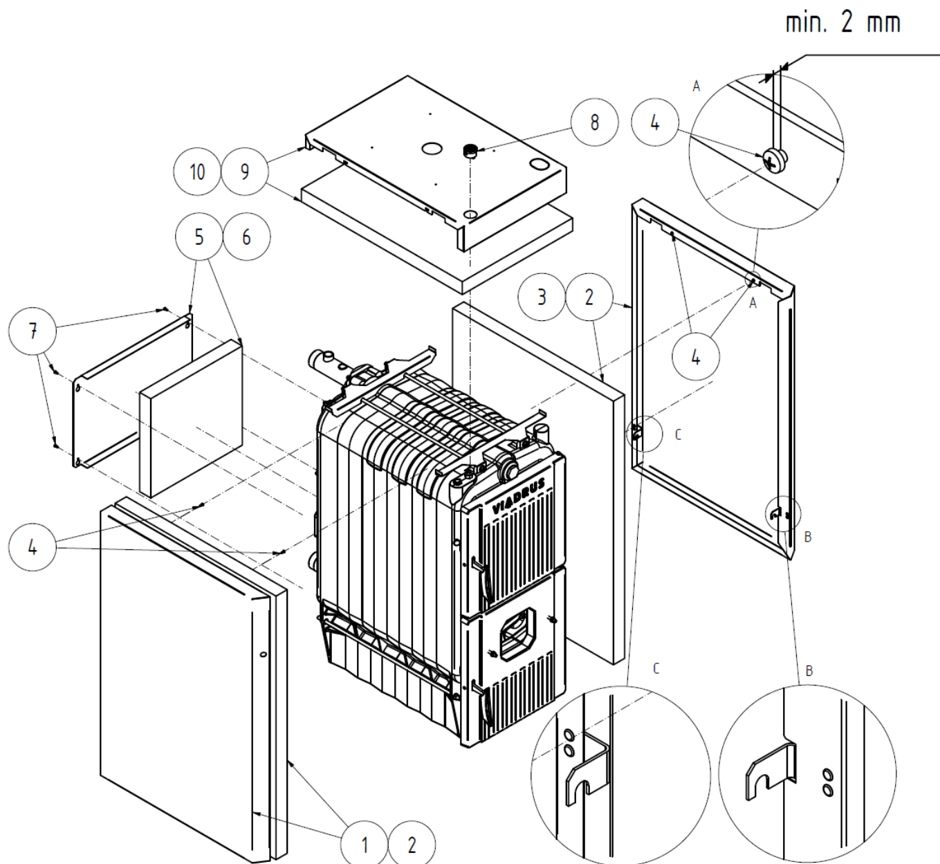
Obr. č. 16 Montáž bočních dílů pláště
